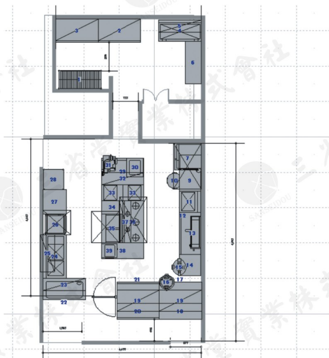
淺草 和食 ふじた 厨房配置図
